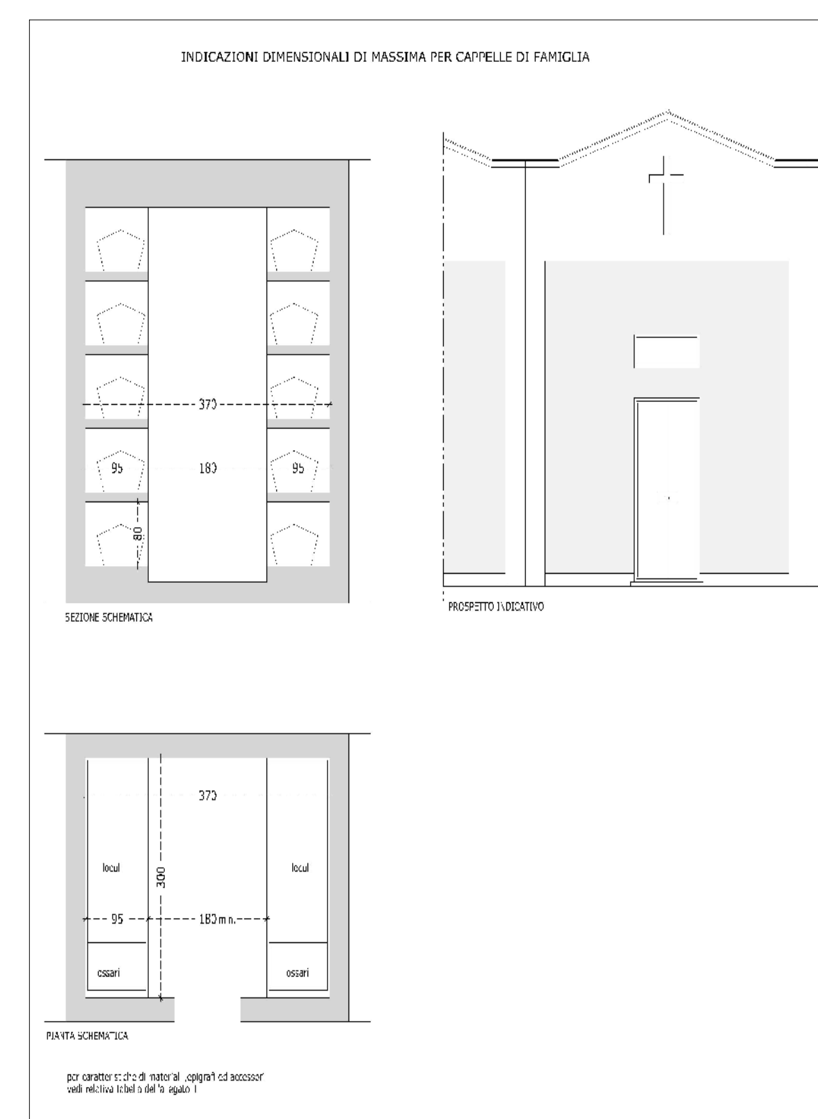
SCHEMA CAPPELLA DI FAMIGLIA
