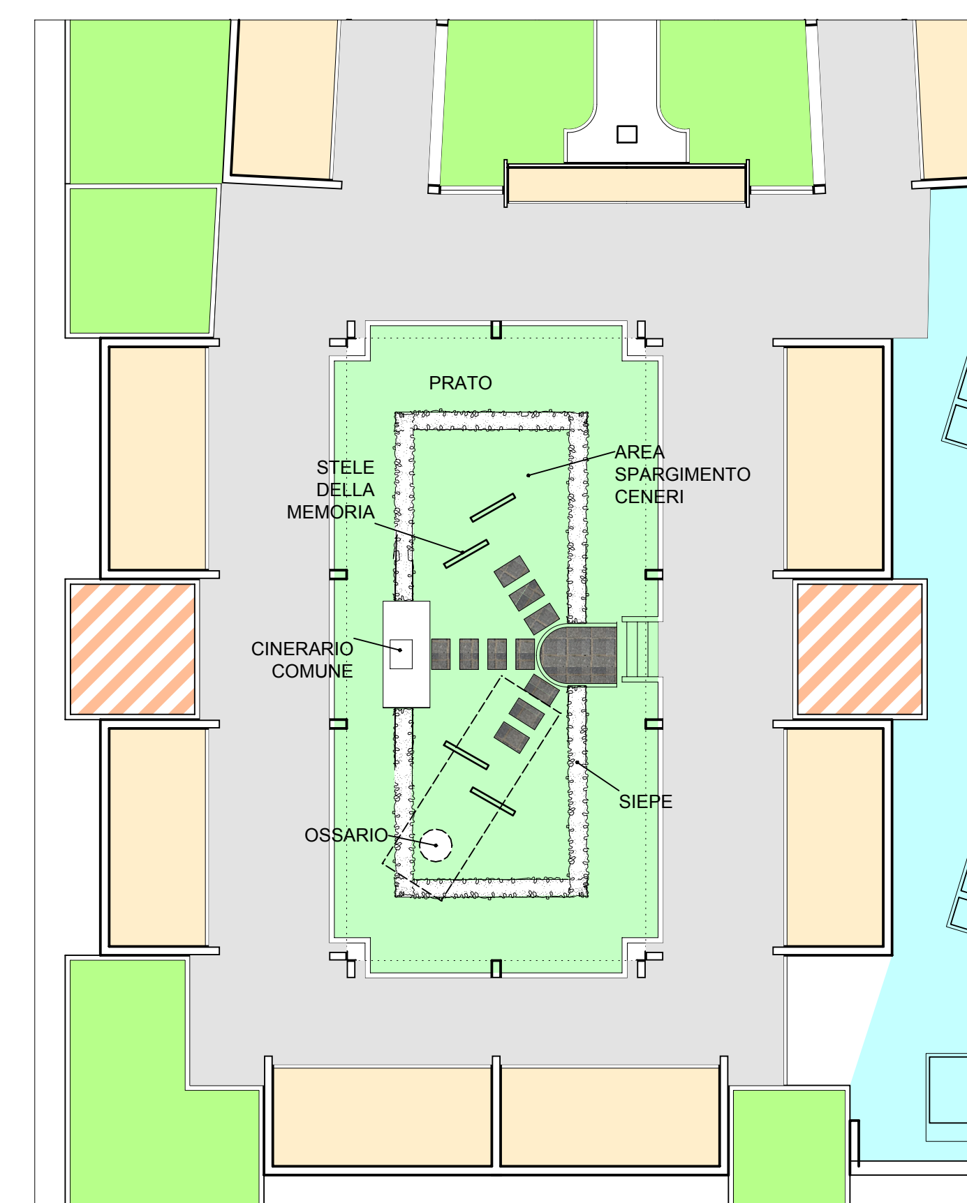
GIARDINO DELLE RIMEMBRANZE scala 1:150
