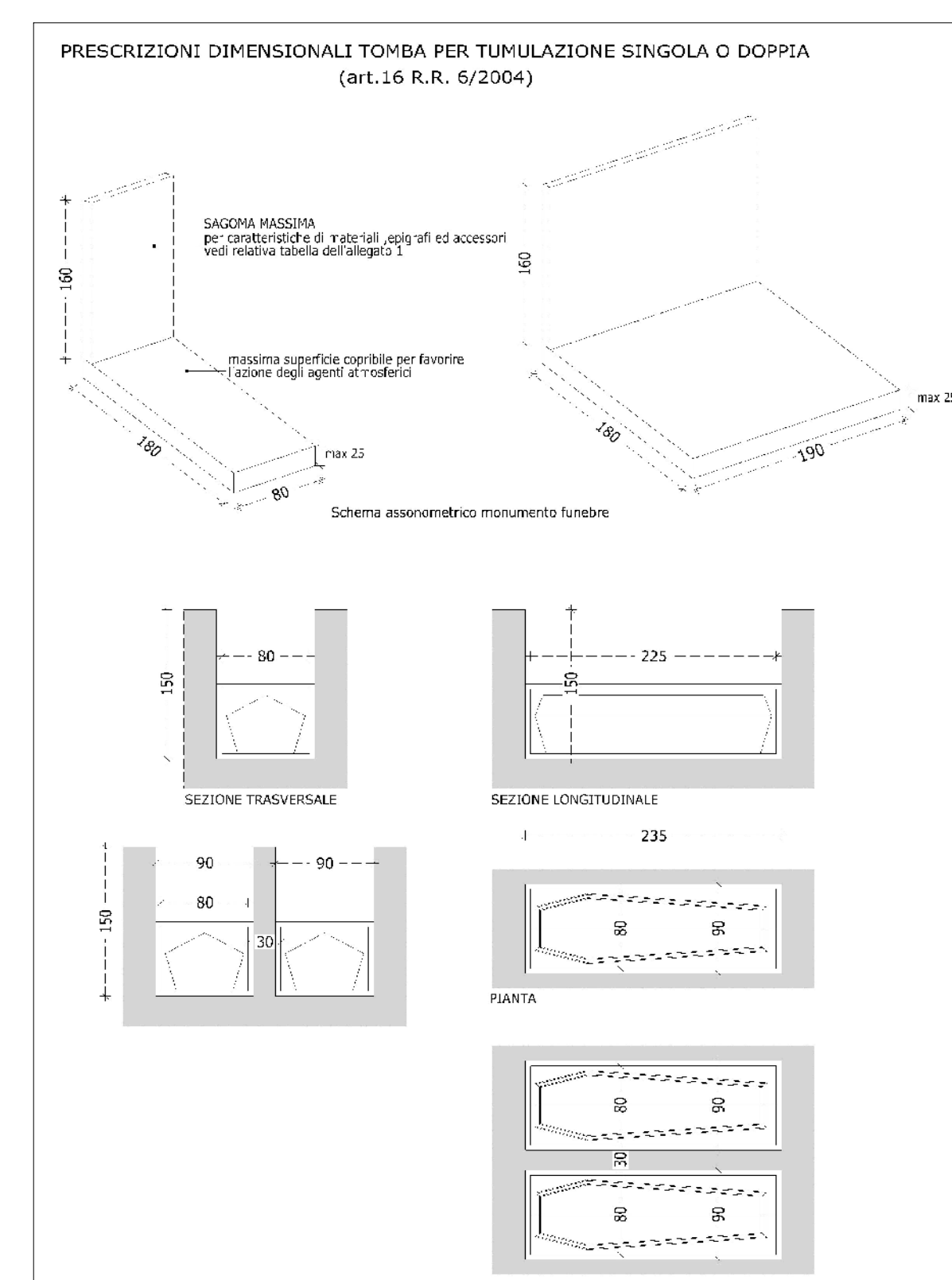
SCHEMA TUMULAZIONI IPOGEE
